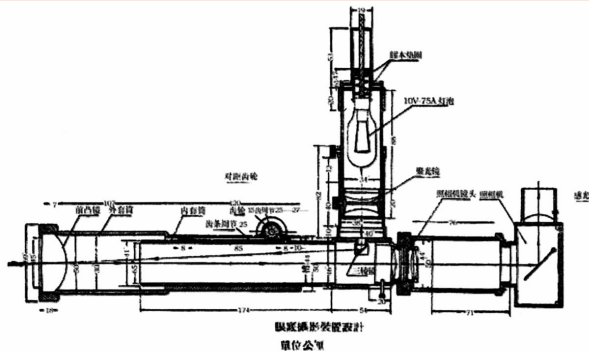
陆道炎研制的眼底摄影机示意图(发表于1956年《中华眼科医学杂志》)
