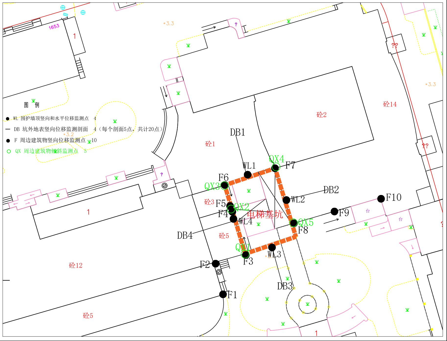
1号楼竖向交通系统改造装饰装修项目基础施工期间监测点布置示意图
